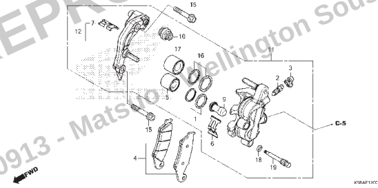
C-12 Cáliper do Freio Dianteiro
