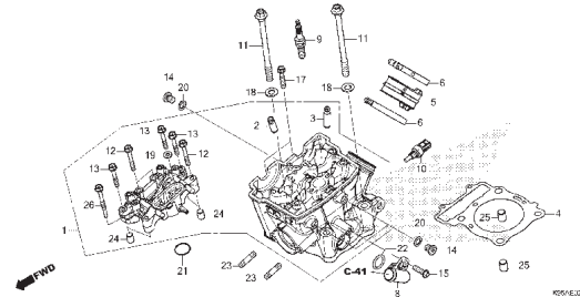
M-5 Cilindro
