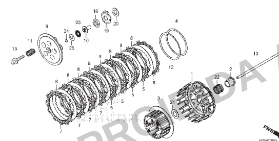
M-8 Embreagem
