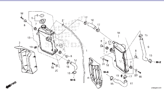
C-41 Radiador
