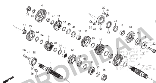
M-17 Transmissão
