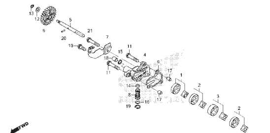
M-16.10 Balanceiro
