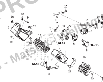
C-37 Bateria
